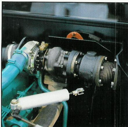
Den nya turbon ger motorn ännu bättre dragkraft på låga varv.
