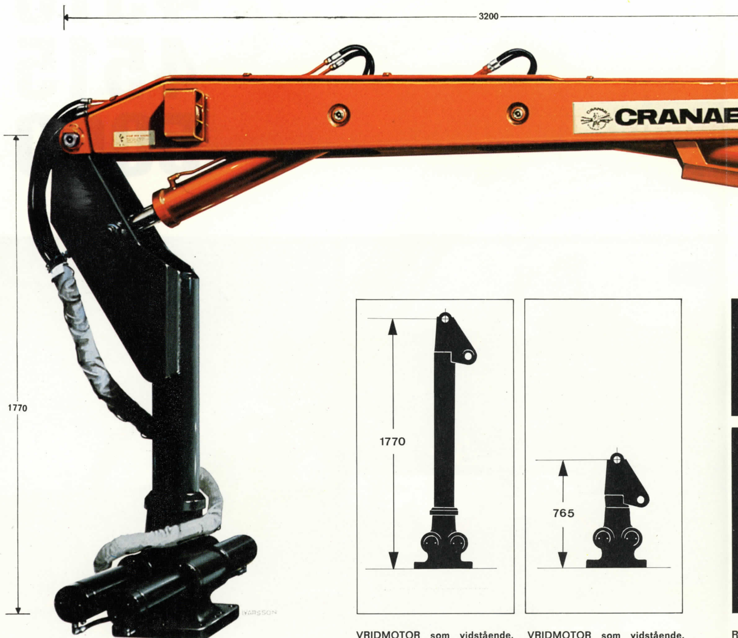
VRIDMOTOR som vidstående, men med rak kranstomme.
